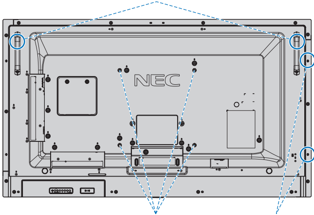
Interfaz de montaje VESA (M6) Cable de seguridad para instalación en vertical
