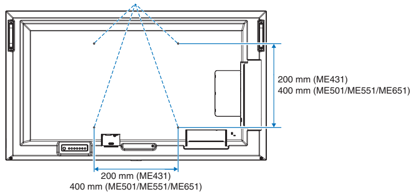
Interfaz de montaje VESA M6 (ME431/ME501/ME551), M8 (ME651)
